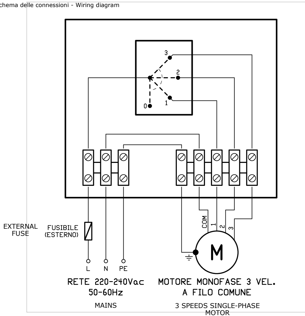
Fig.1/Pic.1 Schema delle connessioni - Wiring diagram
